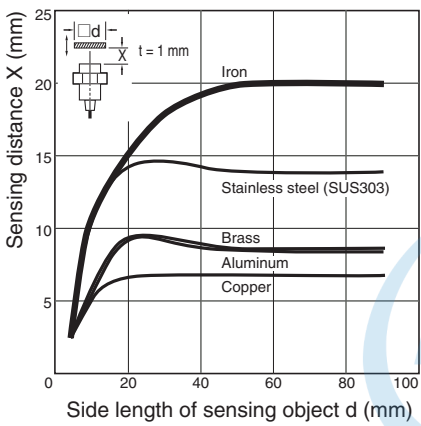
E2A-M30KN20
