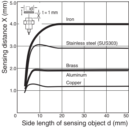
E2A-S08□N04/M08□N04
