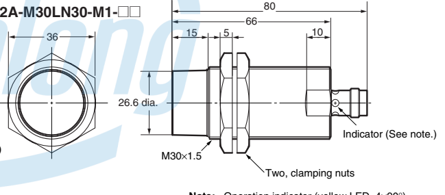
E2A-M30LN30-M1-□□
