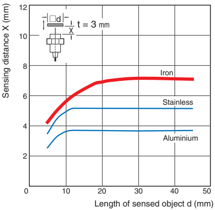
E2NC-EM07M(-□)
