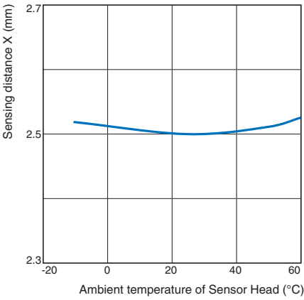
E2NC-EV05(-□)
