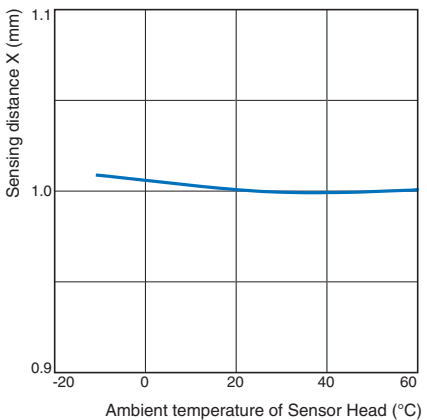
E2NC-EM07M(-□)
