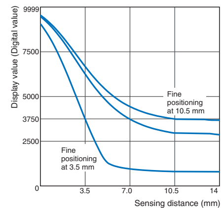
E2NC-EM07M(-□)
