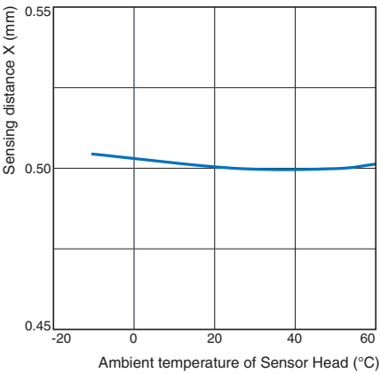
E2NC-EV05(-□)
