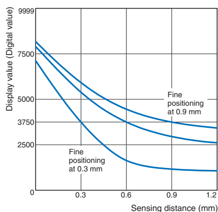
E2NC-EM02(-□)
