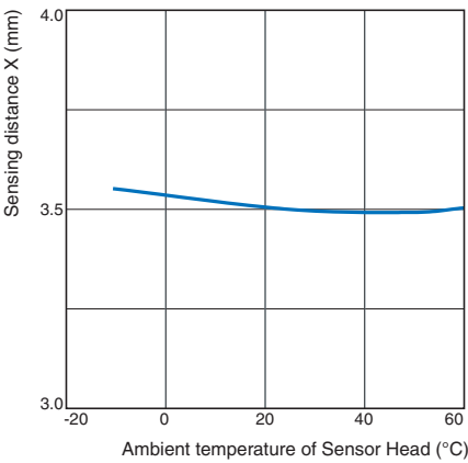
E2NC-EM07M(-□)
