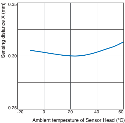
E2NC-EM02(-□)
