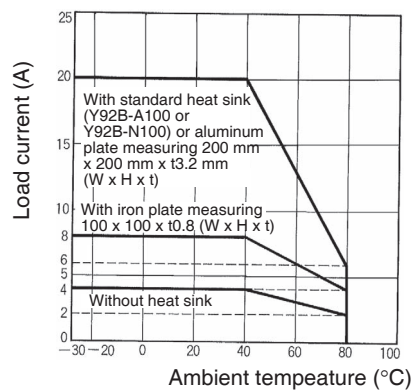
G3NA-440B-UTU-2
