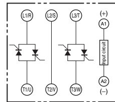
G3PE-515B-2N
