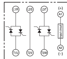
G3PE-535B-2N
