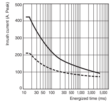
G3PE-535B(L), G3PE-545B(L)
