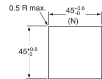
Mounting Hole Dimensions (Conform to DIN 43700.)
